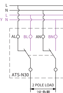
ATS-N30 主回路2P接線圖
