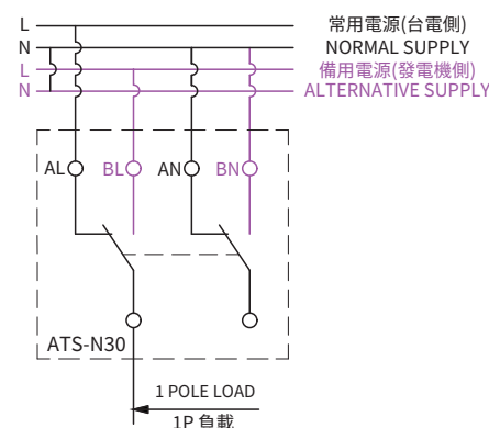
ATS-N30 主回路1P接線圖
