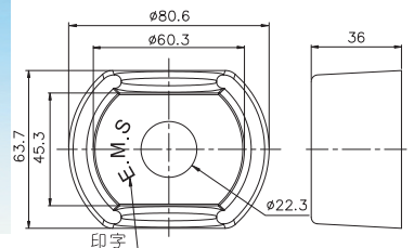
TN2-EA (連鎖式護座無印字) TN2-EB (連鎖式護座)
