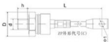
ZP 600A尺寸
