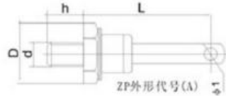
ZP外形代号(A)
