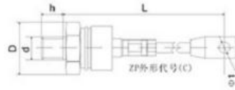
ZP 100A尺寸
