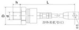
ZP 50A尺寸
