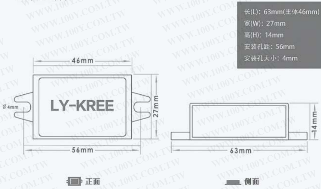
瑞 平面尺寸图
