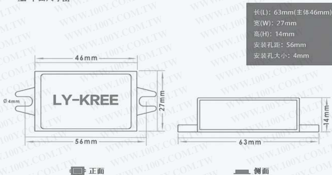
五 平面尺寸图
