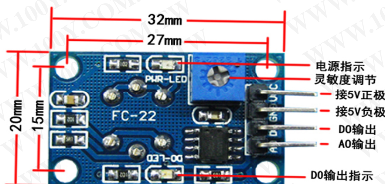
接线图
