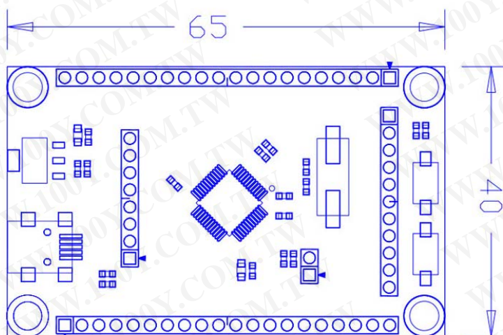
产品结构
