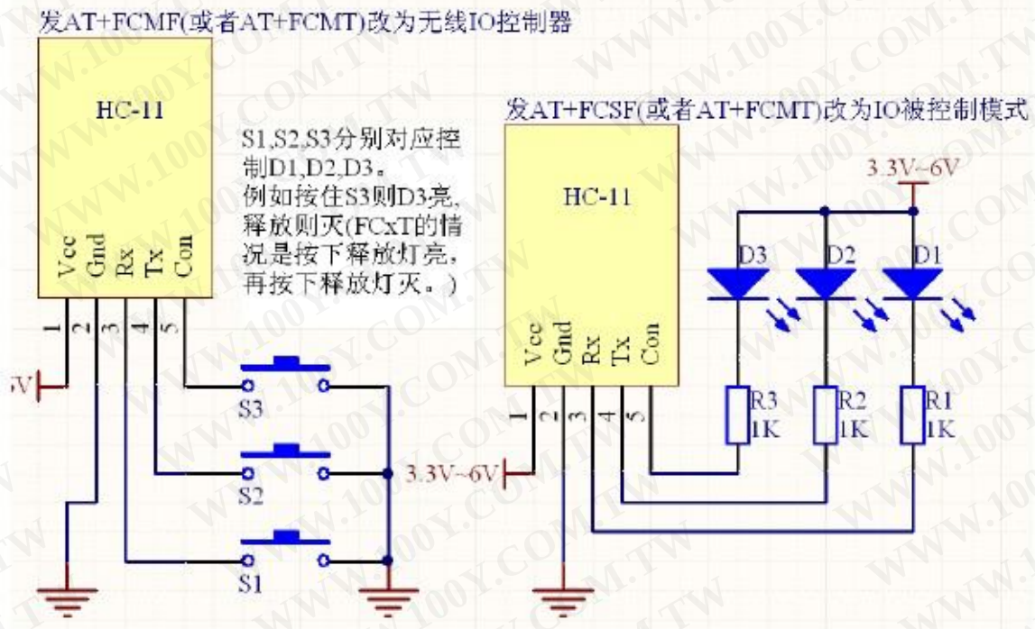
图四、无线 IO 控制的简单试验
