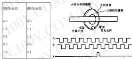
图 3 光电编码器工作原理图及输出波形
