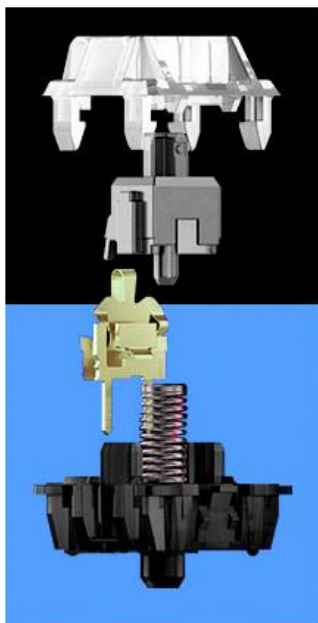
轴体结构拆解图
