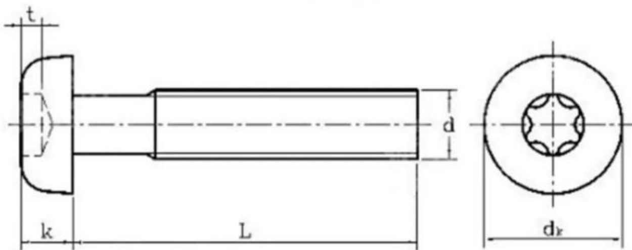
测量示意图
