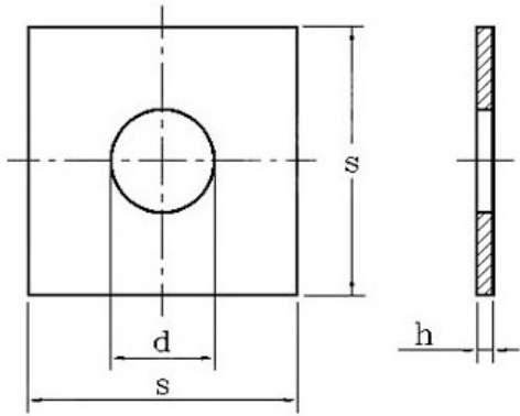
测量示意图
