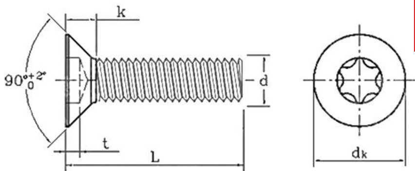
螺丝测量示意图
