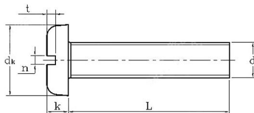
测量示意图
