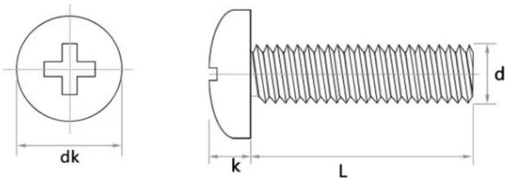
测量示意图
