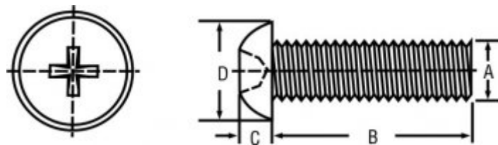
十字圓柱頭塑料螺絲緊固件工程圖
