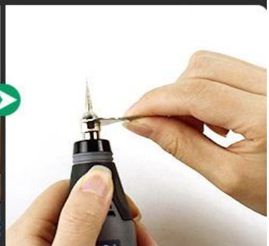
按下锁轴键用扳手顺时针把夹头拧紧固定
