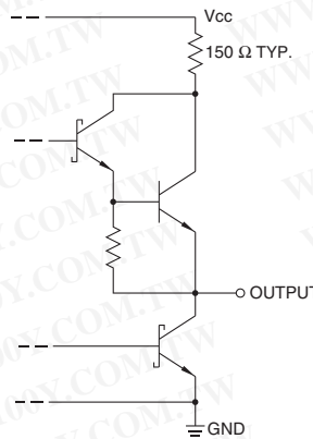
74OL6000/01 Output
