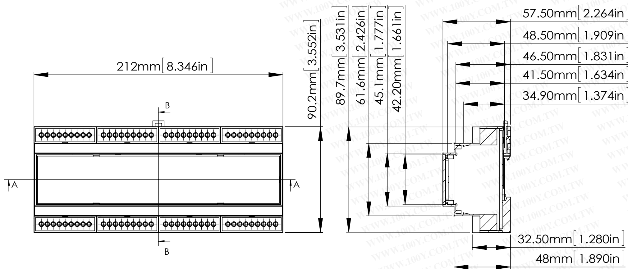
SECTION A-A
