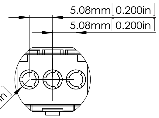
SECTION D SCALE 2 : 1
