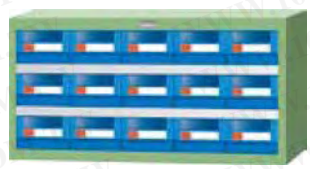
RM-515 H468xW900xD420 抽屨材質：ABS+PS 抽屨配置：TR-4116零件盒15 pcs
