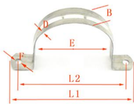
规格举例: 例如 φ8 管卡圈内直径8mm
