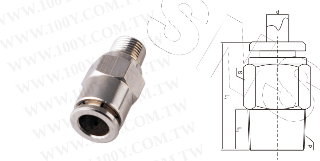
JPC系列-螺纹直通
