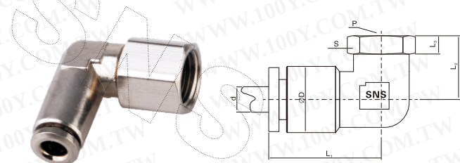
JPLF系列-弯头内螺纹
