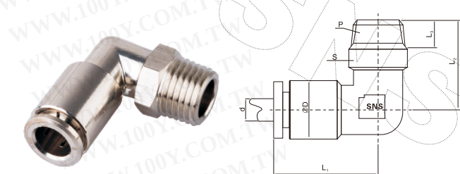
JPL系列-螺纹弯通
