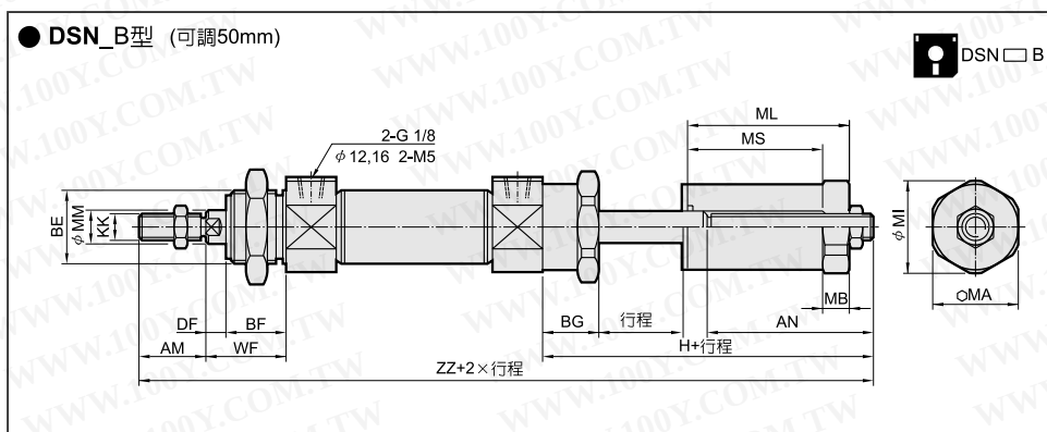
外形尺寸表
