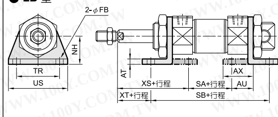
外形尺寸表
