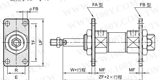
外形尺寸表
