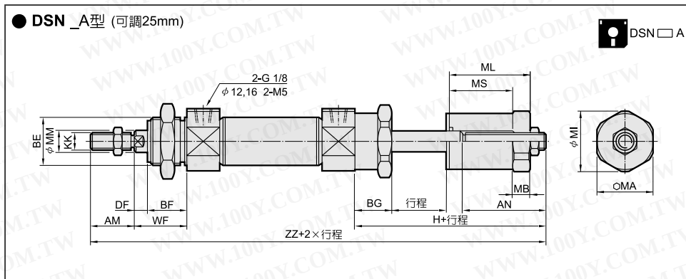
外形尺寸表
