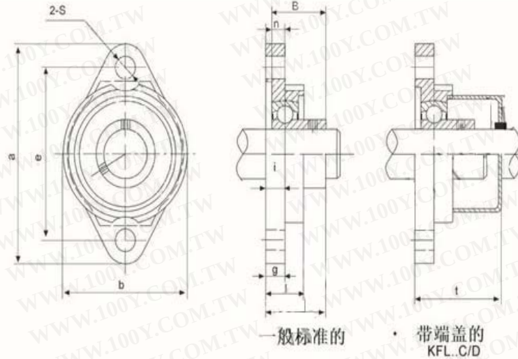
KFL000系列 Two-BOLT FALANGE UNITS
