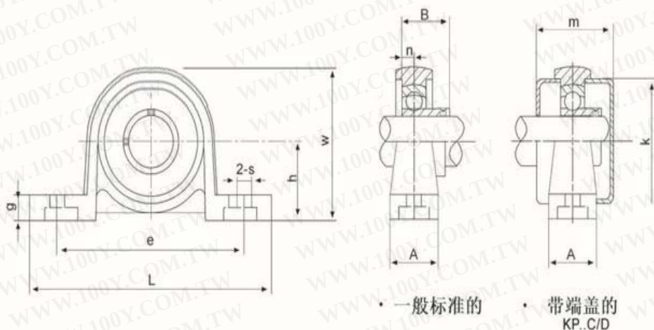
KP000系列 PILLOW BLOCKS
