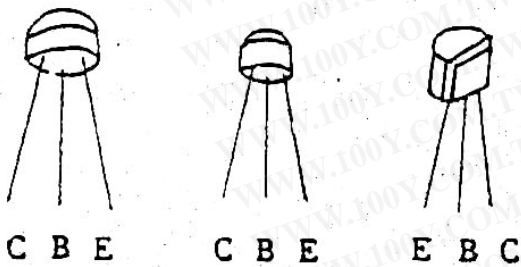
晶體接腳圖
