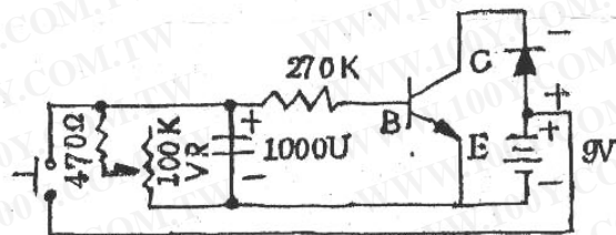
線路圖
