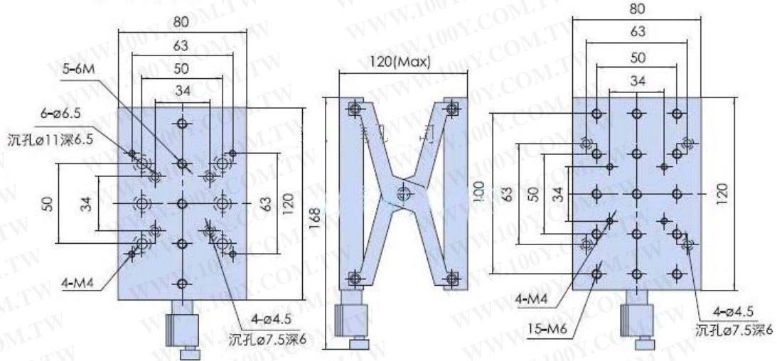
PT-SD408【60行程】产品尺寸图:
