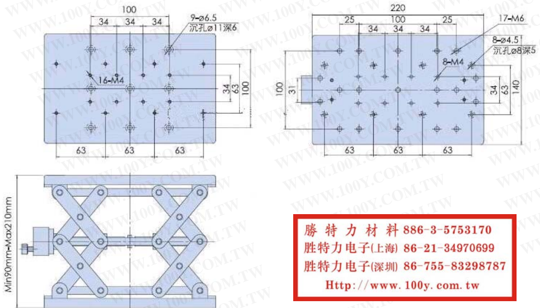
PT-SD409【120行程】产品尺寸图:
