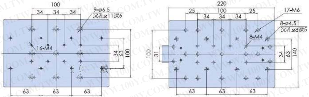
PT-SD409【120行程】产品尺寸图:
