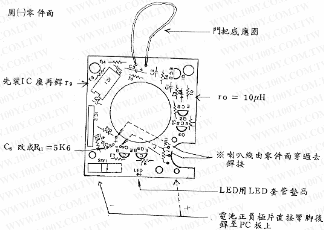
圖(二)銲接面
