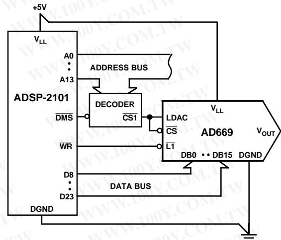
a. ADSP-2101 to AD669 Interface
