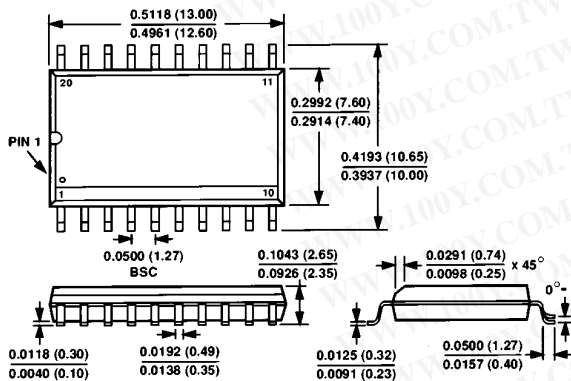
20-Pin SOIC (R-20)
