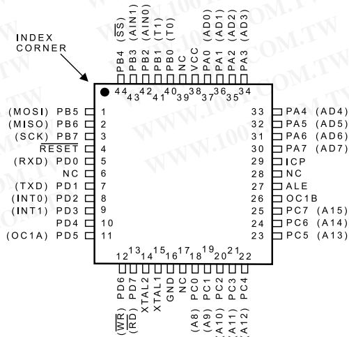
TQFP
