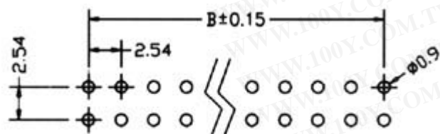
P.C.Board Layout
