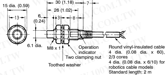
Fig. 4: E2E-X8MD□-N
