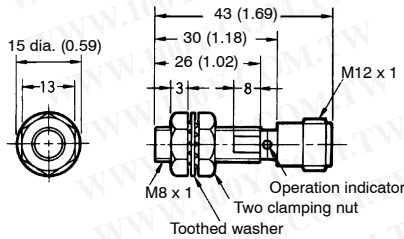
Fig. 9: E2E-X2D□-M1G-N
