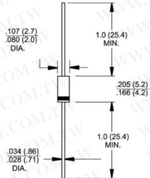
DO-204AL (DO-41)
