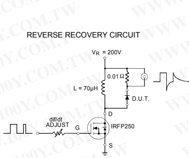
Fig. 9 - Reverse Recovery Parameter Test Circuit
