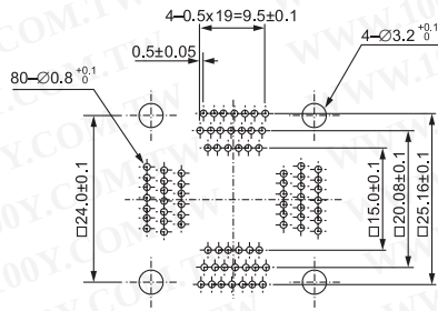
IC51-0804-711 (80 Pins)
