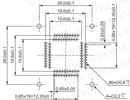
IC51-0804-956-2 (80 Pins)
