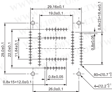
IC51-819-KS12720 (80 Pins)
