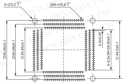
IC51-2404-1655-3 (240 Pins)
