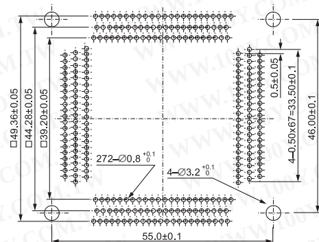
IC51-3044-1471-2 (304 Pins)
