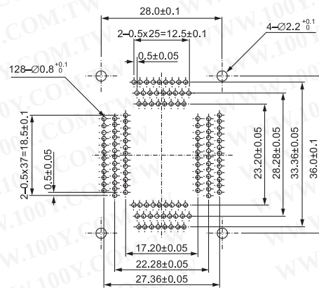
IC51-1284-844-1 (128 Pins) IC51-1284-976-1 (128 Pins) IC51-1284-976-2 (128 Pins) IC51-844-KS13329 (128 Pins)
