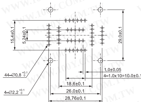
IC51-0444-615 (44 Pins)
