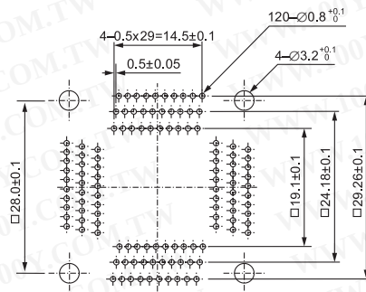
IC51-1204-1652 (120 Pins)
