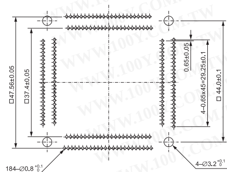
IC51-1844-1541 (184 Pins)
