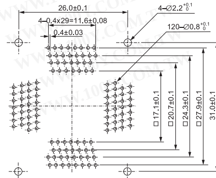
IC51-1204-1812 (120 Pins)
