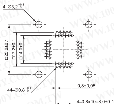
IC51-467-KS11787 (44 Pins)
