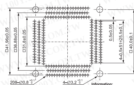
IC51-2084-1052-* 2 (208 Pins)
