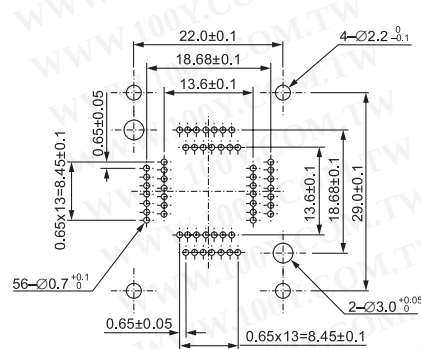
IC51-0564-680 (56 Pins)
