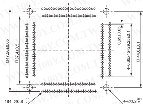
IC51-1844-1148-1 (184 Pins)
