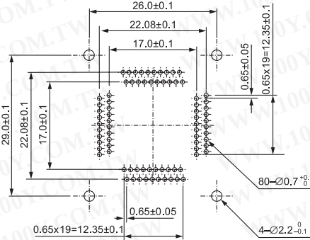
IC51-0804-795 (80 Pins)
