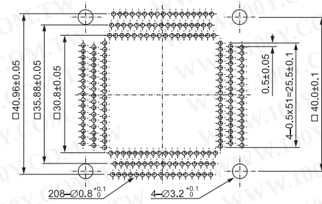
IC51-2084-1509 (208 Pins)
