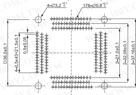
IC51-1764-1505 (176 Pins)
