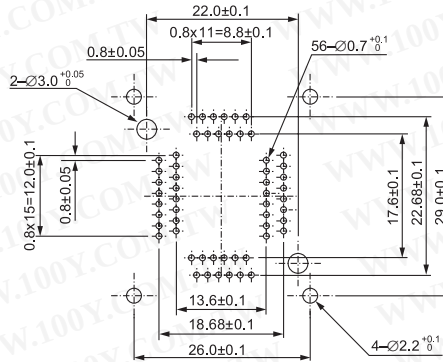
IC51-0564-924 (56 Pins)
