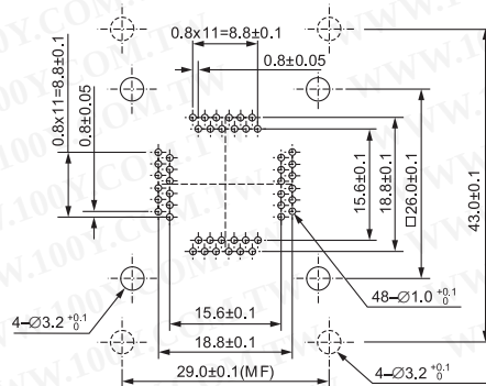
IC51-0484-081 (48 Pins)
