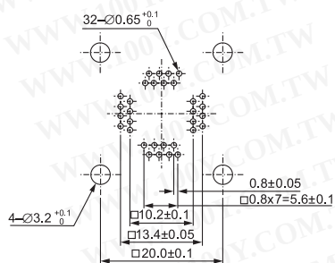
IC51-0324-354 (32 Pins)
