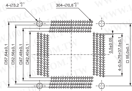
IC51-3044-1471-5 (304 Pins)
