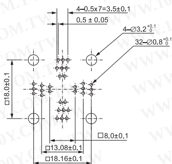
IC51-0324-805 (32 Pins)
