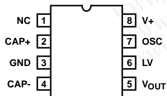
ICL7660, ICL7660A (PDIP, SOIC) TOP VIEW
