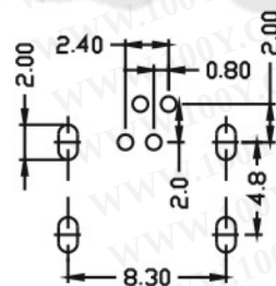
P.C.B LAYOUT
