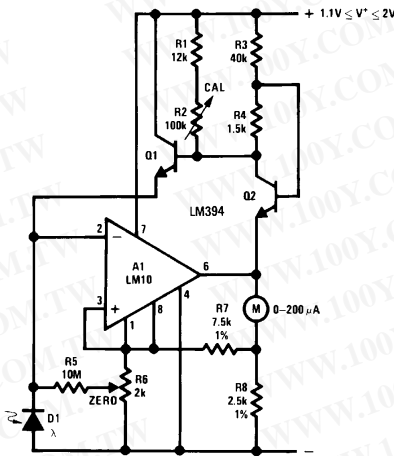
Light Meter
