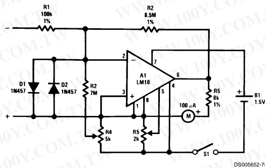
Meter Amplifier
