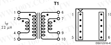
FIGURE 29. Schott 67141450
