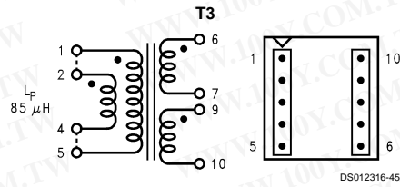
FIGURE 31. Schott 67140920
