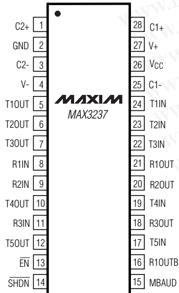
SSOP
