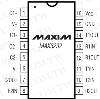
DIP/SO/TSSOP
