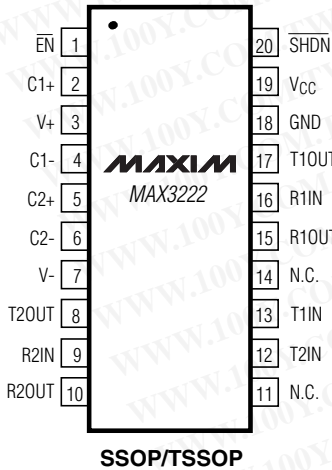
SSOP/TSSOP
