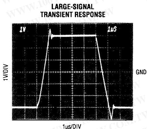
A_v = +1 , R_F = 499\Omega , R_L = 2k\Omega \parallel 20pF V_S = \pm 5V , T_A = +25^\circ C
