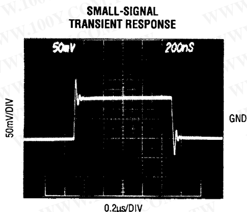
A_v = +1 , R_F = 200\Omega , R_L = 2k\Omega \parallel 20pF V_S = \pm 5V , T_A = +25^\circ C
