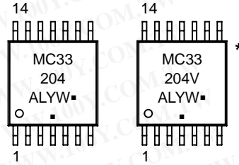
TSSOP-14 DTB SUFFIX CASE 948G
