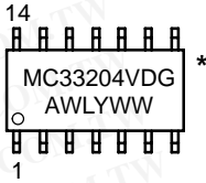
SO-14 VD SUFFIX CASE 751A
