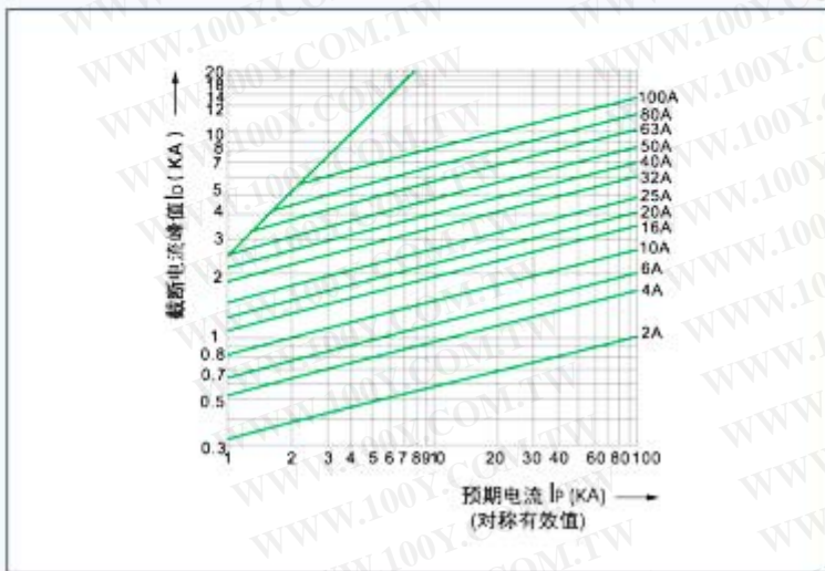
gG 熔断体的截断电流特性
