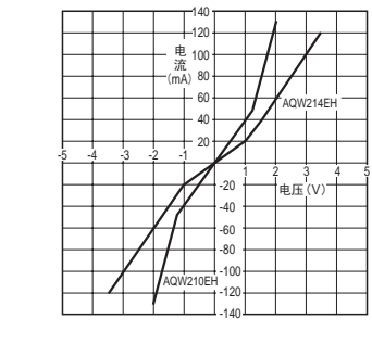
8. - (1) 输出部电流-电压特性 测定位置: 5-6端子间, 7-8端子间 环境温度: 25^{\circ}\text{C}
