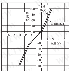
8. 输出部电流—电压特性 测定位置：5-6, 7-8端子间 环境温度：25℃
