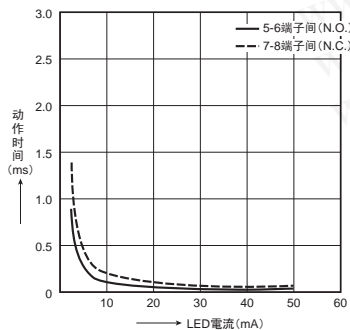
10. 动作时间—LED电流特性 测定位置：5-6, 7-8端子间, 负载电压：400V (DC) 连续负载电流：100mA (DC), 环境温度：25℃
