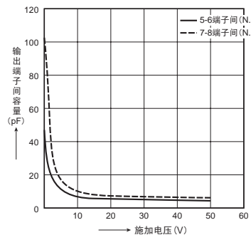
12. 输出端子间容量—施加电压特性 测定位置：5-6, 7-8端子间 频率：1MHz, 环境温度：25℃
