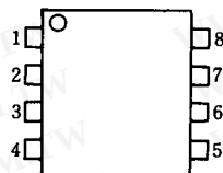
NJM2360D NJM2360M
