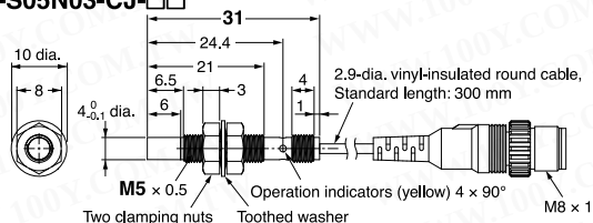
E2E-S05N03-CJ-□□
