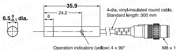
E2E-S05N03-CJ-□□
