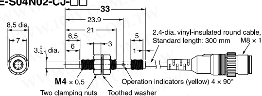
E2E-S04N02-CJ-□□
