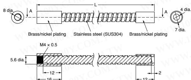
Y92E-ST04-□
